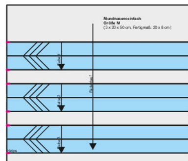
Mundnasenmaske, Schnittteil
